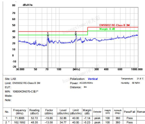
图 5-7 RE 测试垂直方向
