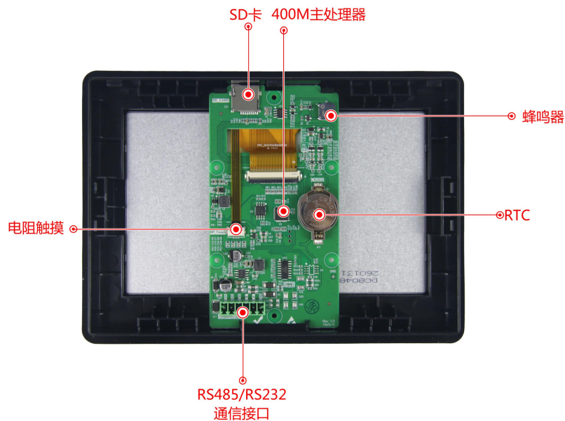
图 1-2 RS232 硬件配置图
