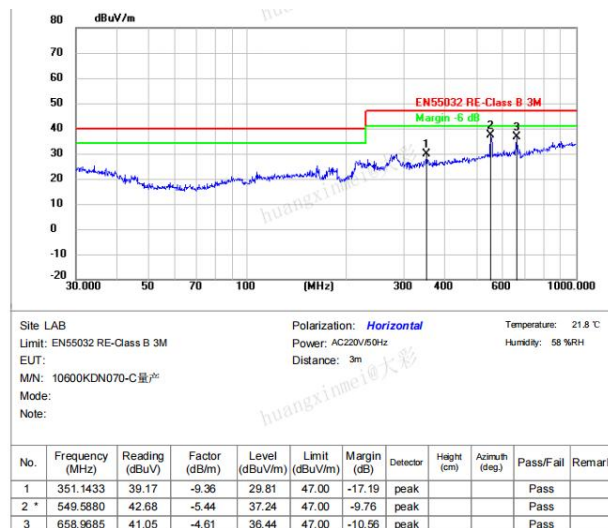
图 5-6 RE 测试水平方向
